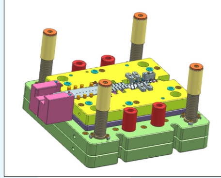
टर्मिनल बॉक्स के लिए प्रगतिशील उपकरण
