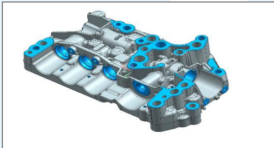
सोलनॉइड बॉडी
