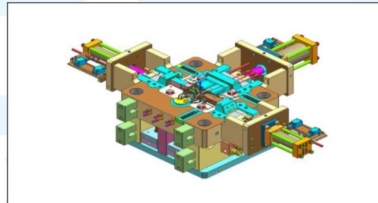
सोलनॉइड बॉडी एचपीडीसी डाई के लिए मूविंग हाफ वाल्व बोडी
