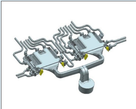
ईसीयू कवर के लिए शॉट मॉडल
