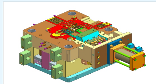
एचपीडीसी डाई के लिए मूविंग हाफ
