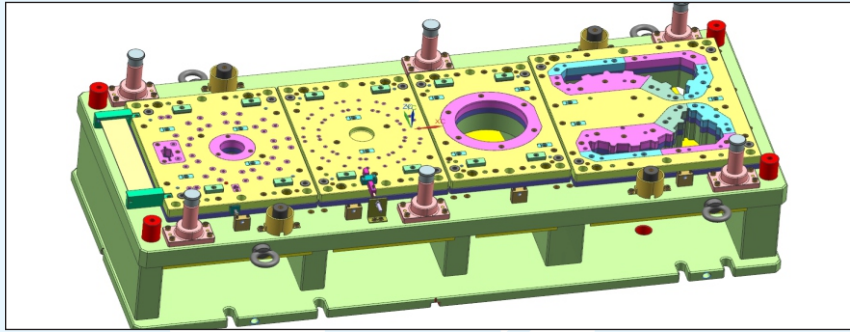
ड्रिवेन प्लेट प्रोग्रेसिव टूल के लिए निचला आधा असेंबली
