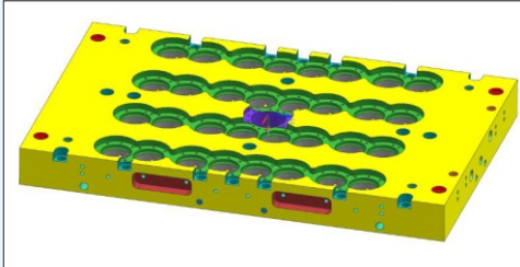
मैनिफोल्ड बैक प्लेट
